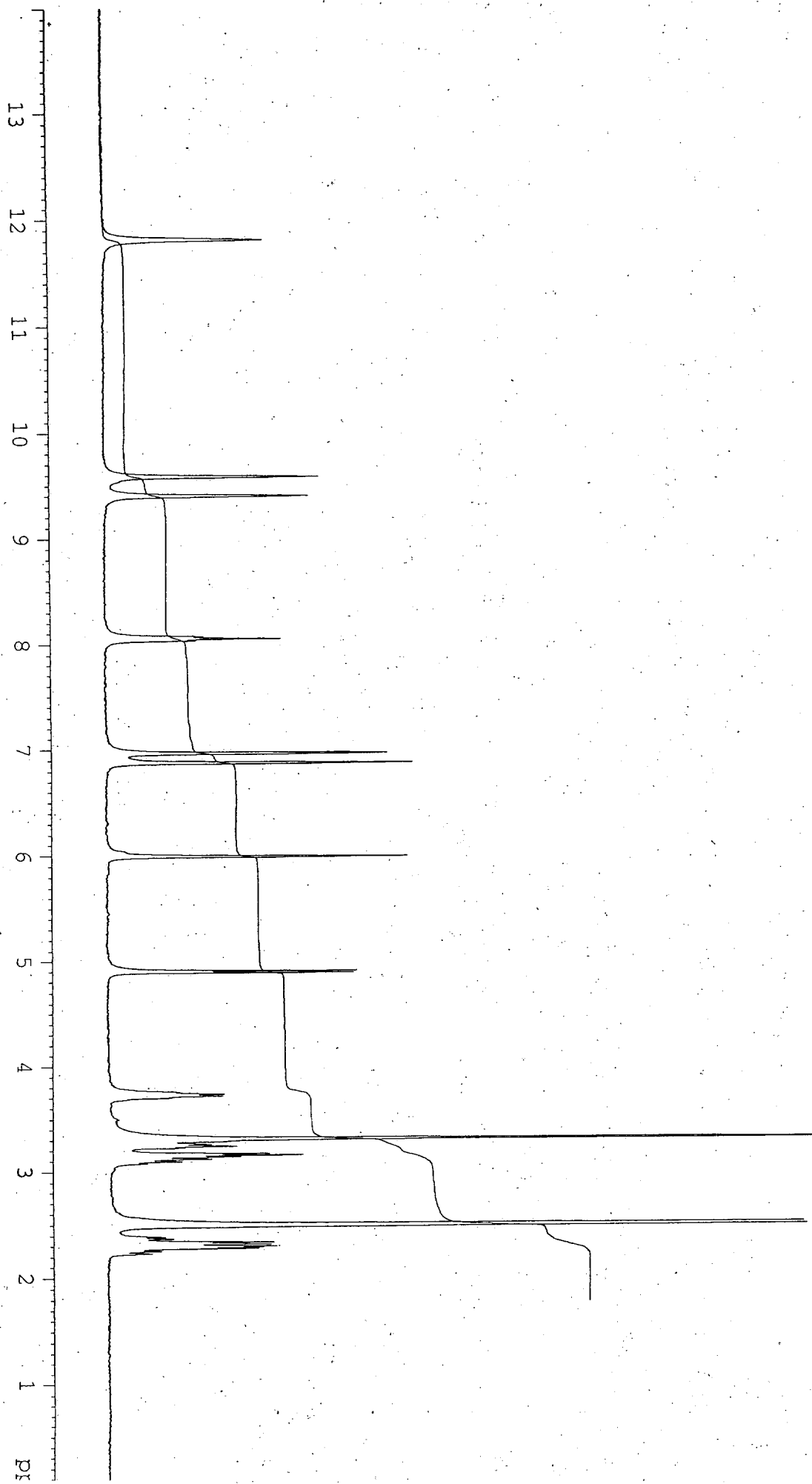
4 DMSO- d 6
