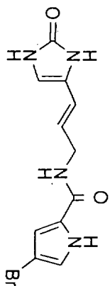
9 DMSO- d 6
