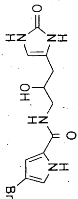
4 DMSO- d 6
